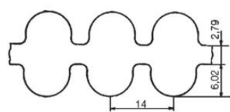
Kuggrem HTD D14M
