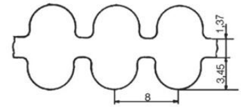
Kuggrem HTD D8M
