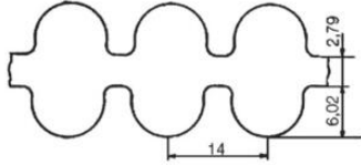
Kuggrem HTD D14M
