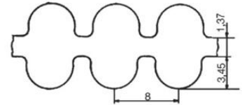
Kuggrem HTD D8M
