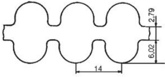
Kuggrem HTD D14M
